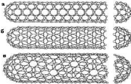
Рис. 2. Класифікація вуглецевих нанотрубок: a – armchair ; б – zigzag ;
