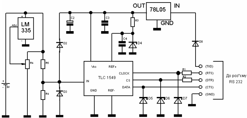
Рис. 2. Принципова схема інтерфейсу для RS232
