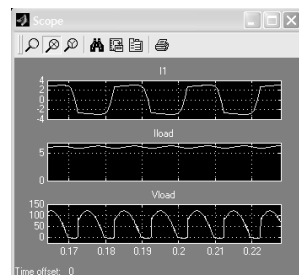
Рис. 11. Осциллограммы тока питания, тока нагрузки и напряжения
