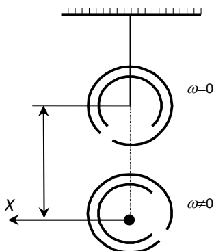
Рис. 1. Схема устройства маятника Максвелла
