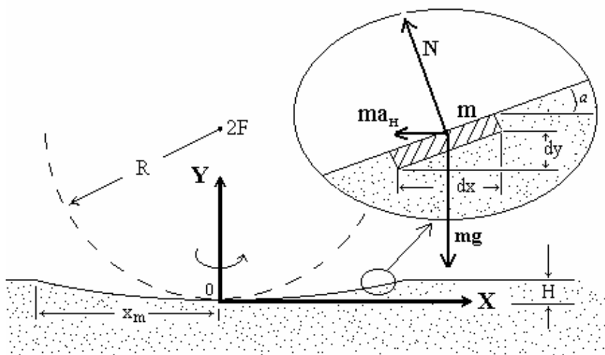
Рис. 2. Характеристики заглибини-дзеркала на поверхні океану
