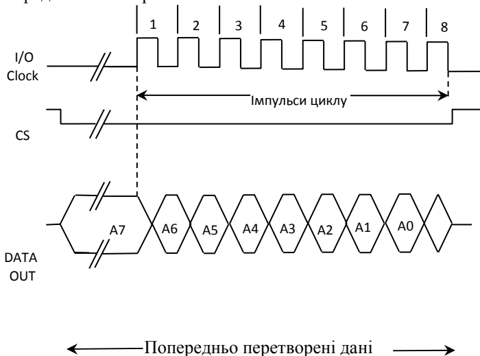
Рис. 3. Протокол зв'язку АЦП TLC 1549IP
