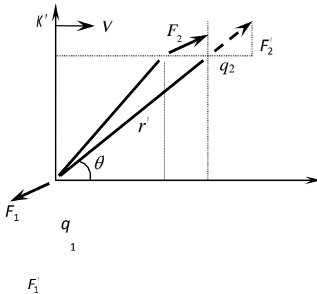
Рис. 6. До обчислення моменту сил, що діють на систему стержень-заряджені частинки [1]
