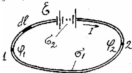
Рис. 2. Електричне замкнене коло: \sigma_1 \sigma_2 – питомі значення електропровідностей однорідної і неоднорідної ділянок кола відповідно
