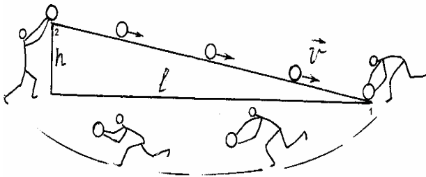
Рис. 3. Неперервний рух м'ячиків по похилій площині під дією сили тяжіння забезпечується “сторонньою силою”, роль якої виконують хлопчики, що переносять скочені м'ячки у верхню частину площини
