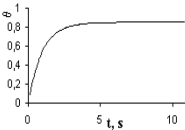
Рис. 1. Розв'язок рівняння (9) з початковою умовою \theta(t = 0) = 0
