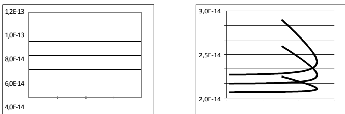
Рис. 3. Траскторії руху \alpha -частинки в досліді Резерфорда
